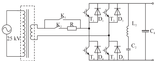
图1 四象限整流器主电路
