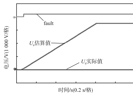
(a)中间直流电压估算
