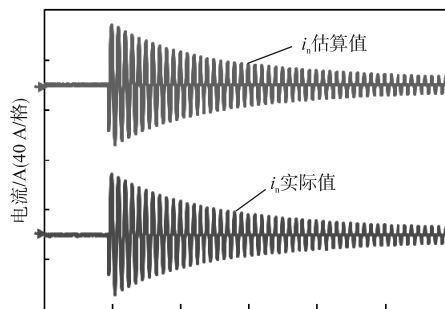
(b)输入电流估算
