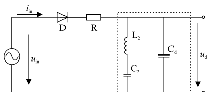
(a)交流电压输入等效电路
