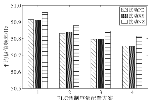
图 16 不同方案的系统平均极值频率
