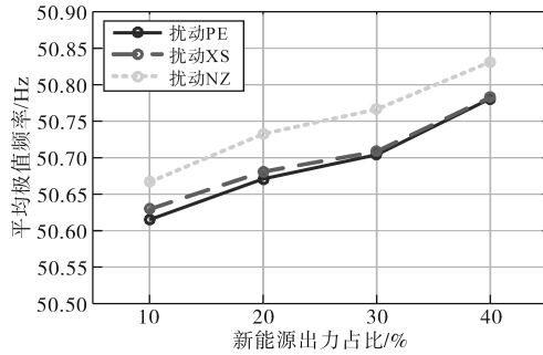
图7 不同新能源出力占比下的系统平均极值频率
