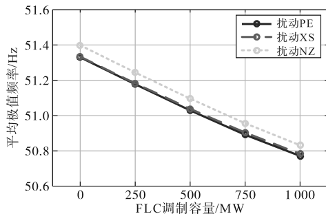
图15 不同直流FLC调节量下的系统平均极值频率
